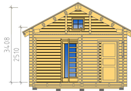
SEKTION A-A
