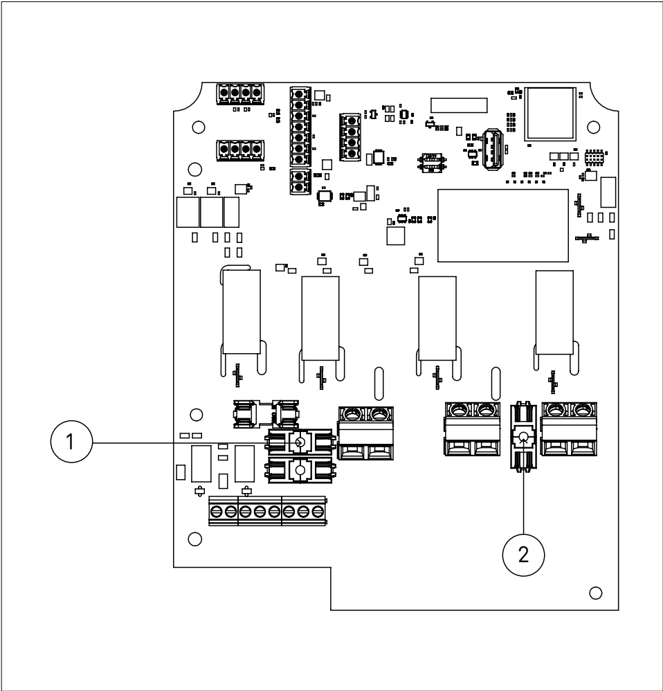
Kuva 5.3-3. Piirikortin lasiputkisulakkeet
