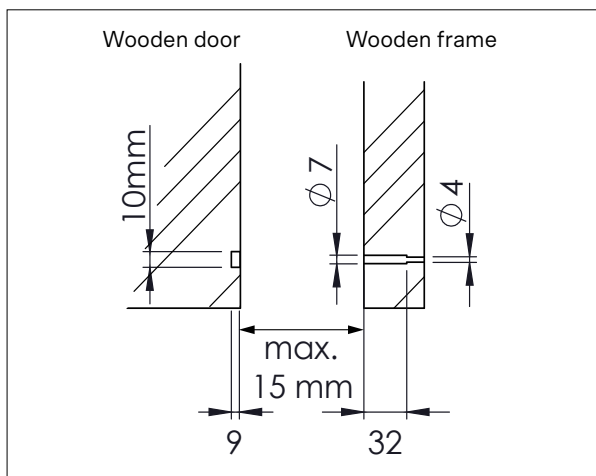
Abbildung 6.7-3: die Einbettung des Türsensors und des Magnetens
