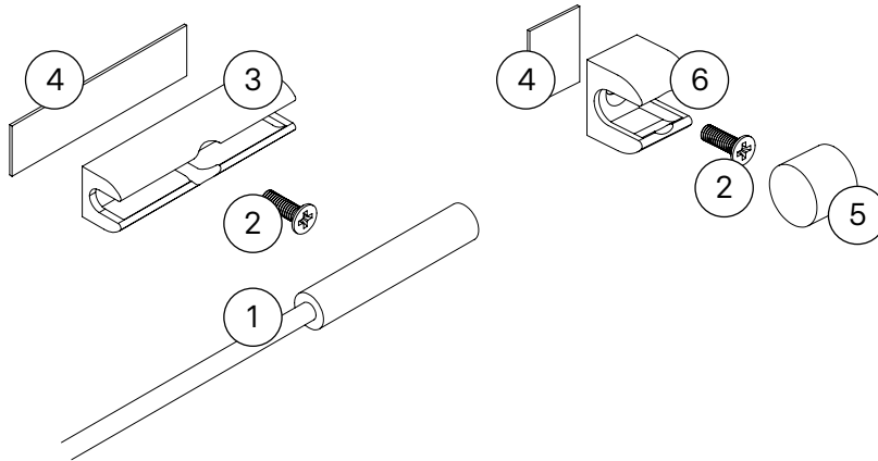
Abbildung 6.7-1: Türsensor einstellen: 1) Türsensor mit Anschlusskabel, 2) Schraube 3) Rahmenswitchhalter 4) Aufkleber 5) Magnet 6) Türmagnethalter
