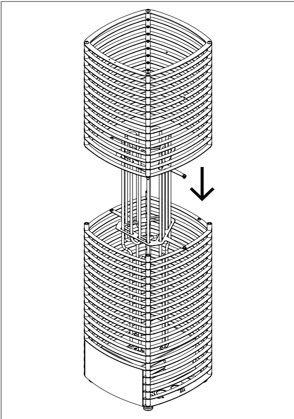
Abbildung 6.9-3: Anbringen des Außengehäuses
