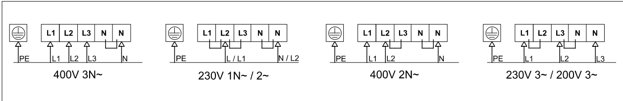
Kuva 5.3-2. Kytentäkaavio E-malli / Flow lisätehoyksiköllä
