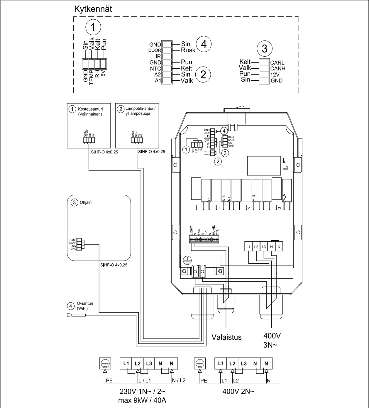
Kuva 5.3-1. Kytkentäkaavio
