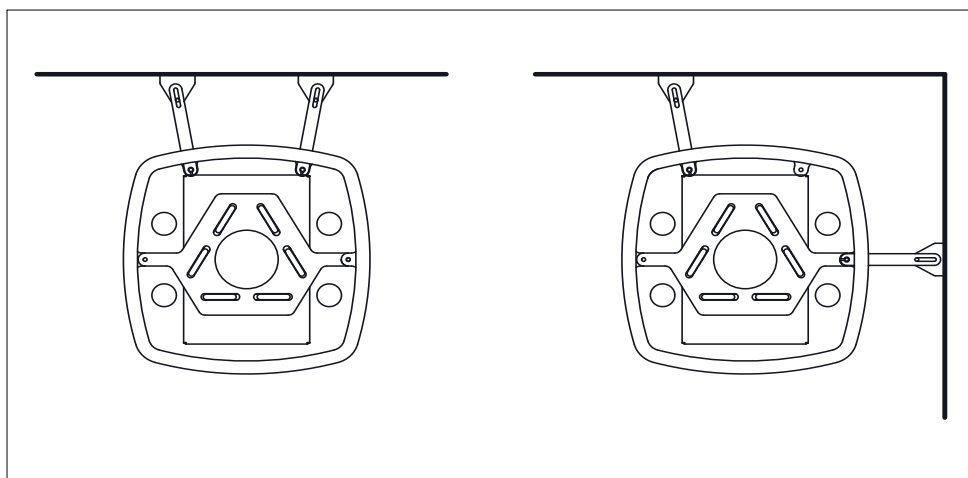
Kuva 6.9-2. Tukirautojen asennus
