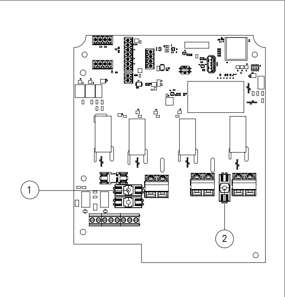
Bild 5.3-3: Kretskortets glasrörssäkringar
