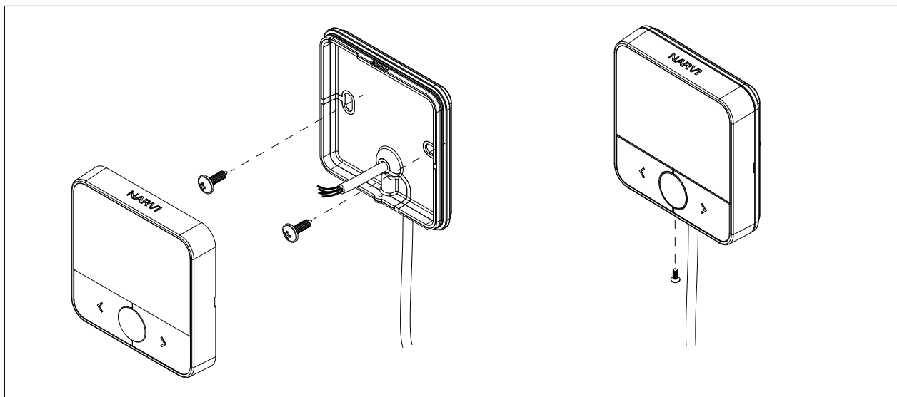
Kuva 6.4-1. Ohjainkotelon asennus
