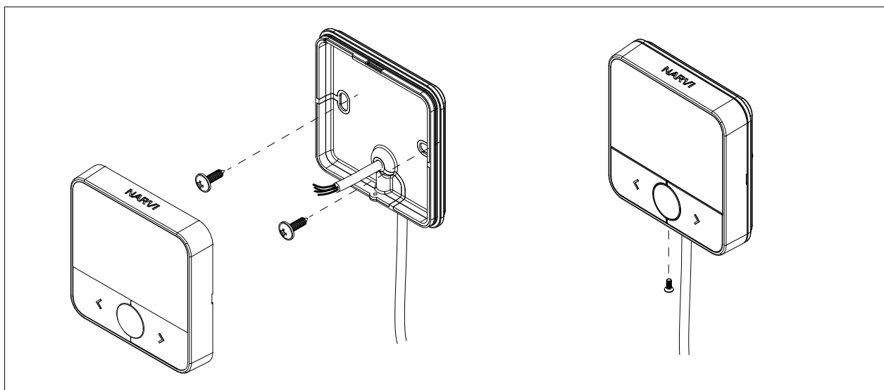
Bild 6.4-1: Installation av styrbox
