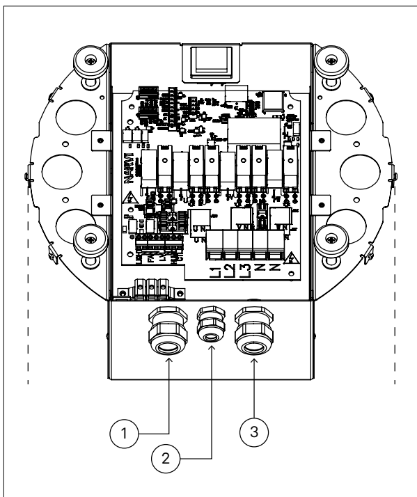
Abbildung 6.3-1: Kabeleinführungen des Anschlusskastens
