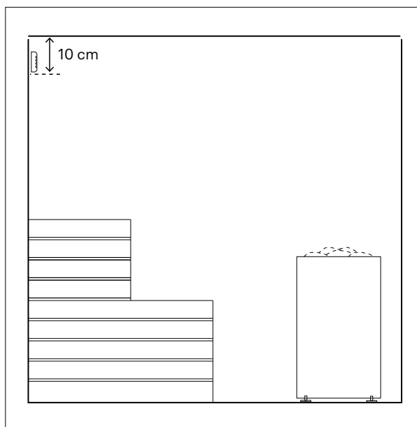
Kuva 6.6-1. Kosteusanturin asennus
