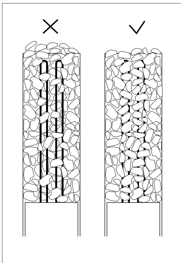
Abbildung 6.9-1: Auflegen der Saunaofensteine
