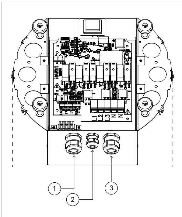
Kuva 6.3-1. Kytkentäkotelon läpiviennit
