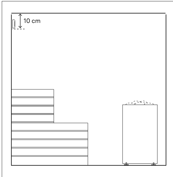
Abbildung 6.6-1: Installation des Feuchtigkeitssensors
