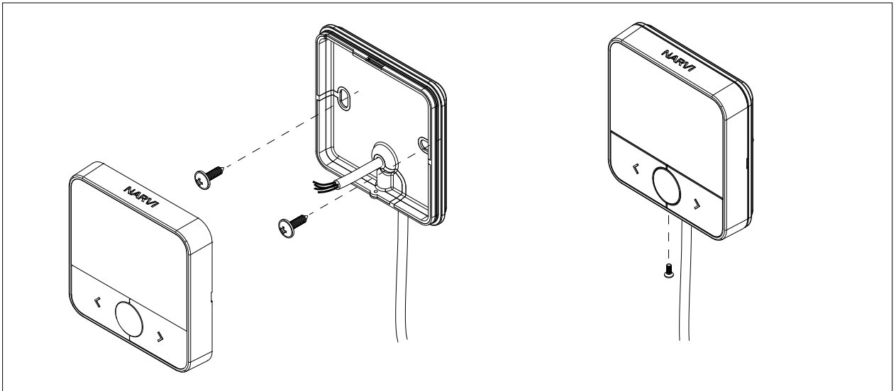
Abbildung 6.4-1: Installation des Gehäuses des Bedienfeldes
