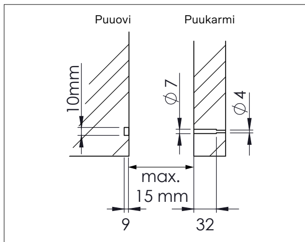
Kuva 6.7-3. Ovikytkimen ja magneetin upotus
