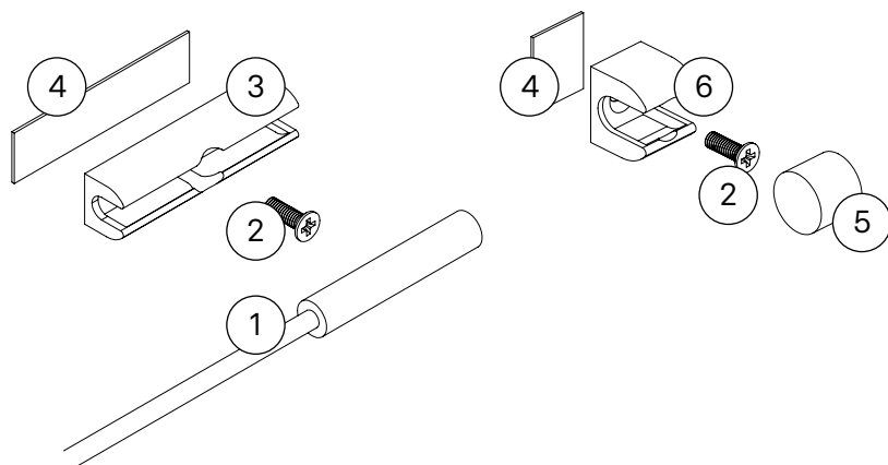
Bild 6.7-1: Dörrkontaktens uppsättning: 1) Dörrkontakt med anslutningskabel, 2) Skruv 3) Fäste för dörramen 4) Klistermärke 5) Magnet 6) Magnetfäste för dörren
