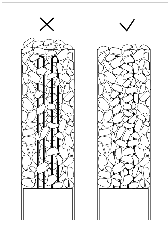
Bild 6.9-1: Stapling av bastustenar
