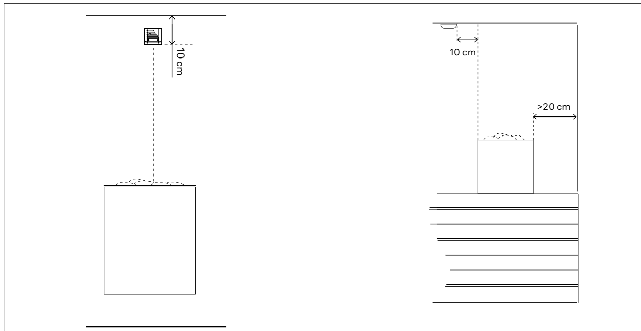
Bild 6.5-1: Installation av temperatursensorn
