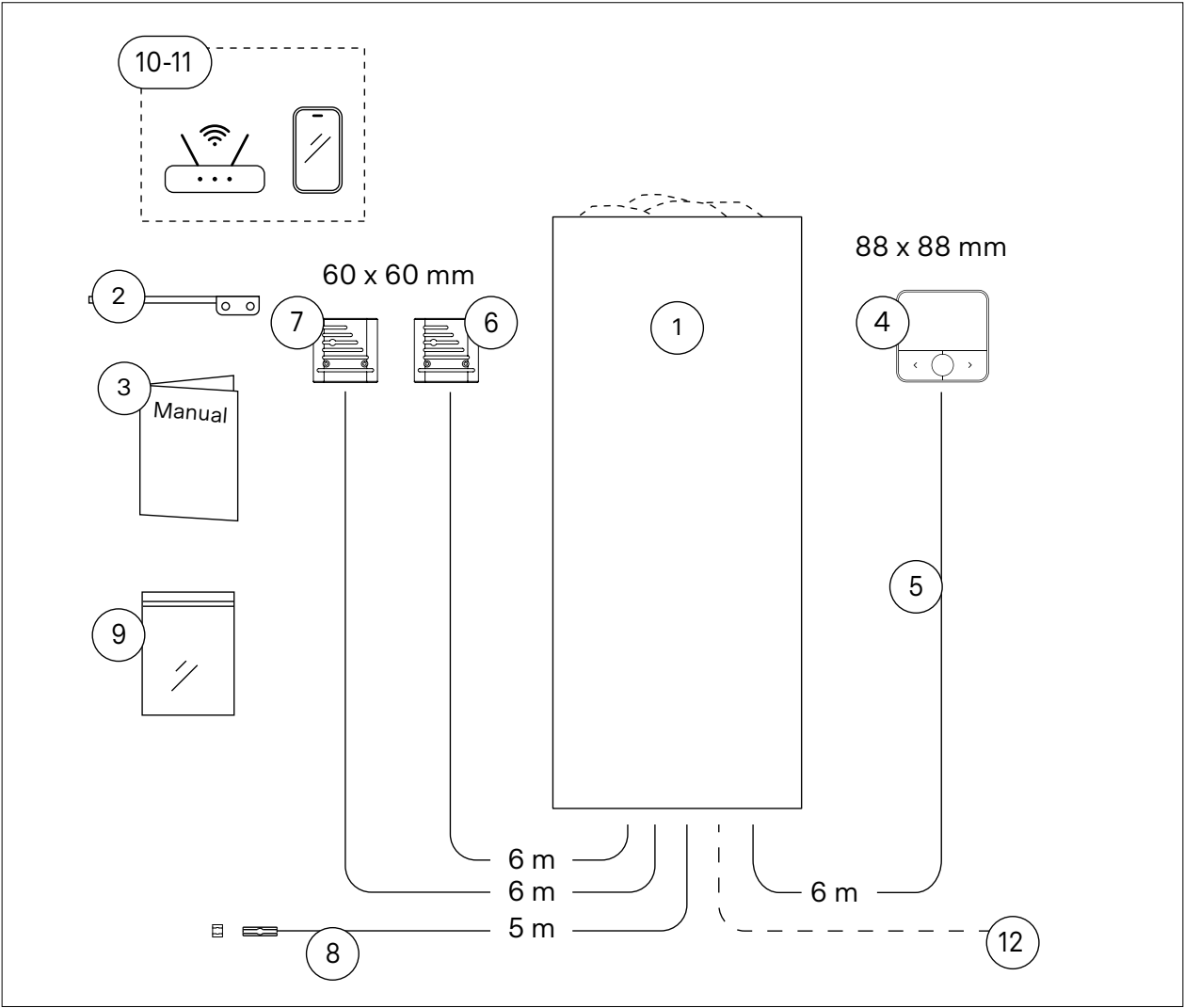
Abbildung 5.1-1: Teile des Systems
