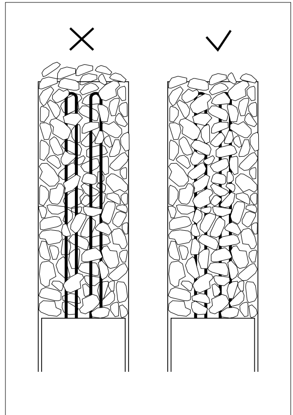
Kuva 6.9-1. Kiuaskivien ladonta
