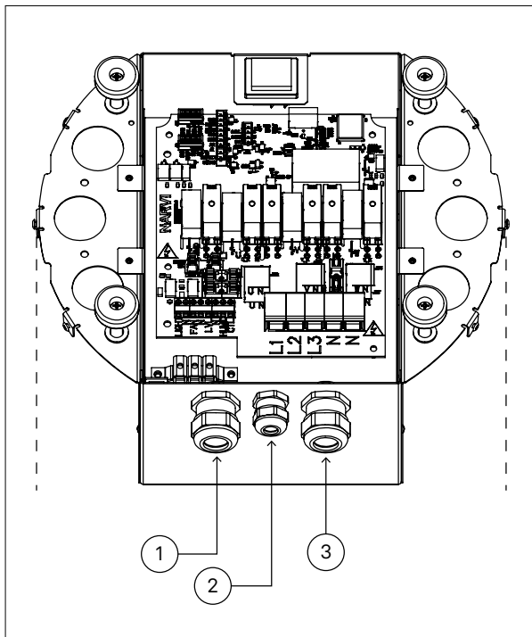
Bild 6.3-1: Kopplingsboxens genomföringar
