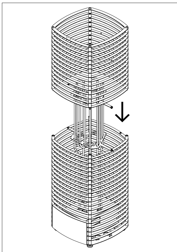
Bild 6.9-3: Montering av ytterhöljet
