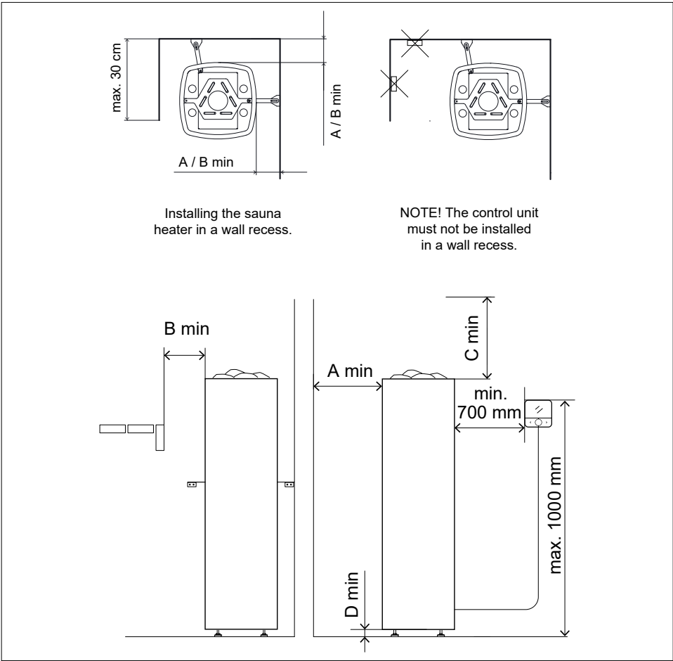
Abbildung 6.1-1: Mindestsicherheitsabstände
