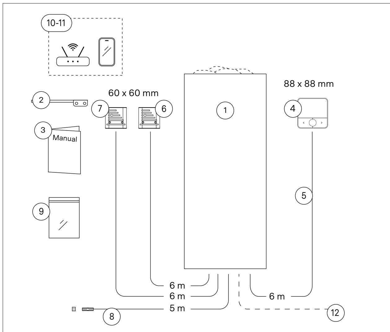
Bild 5.1-1: Bastusystemets delar
