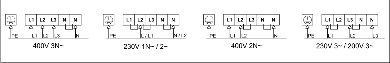
Bild 5.3-2: Kopplingsschema E-modell / Flow med extra effektenhet
